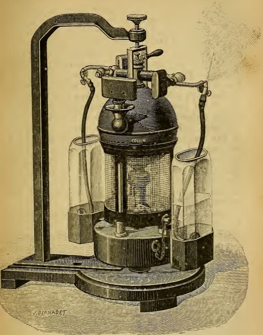
Fig. 35. — Pulvérisateur tournant.
